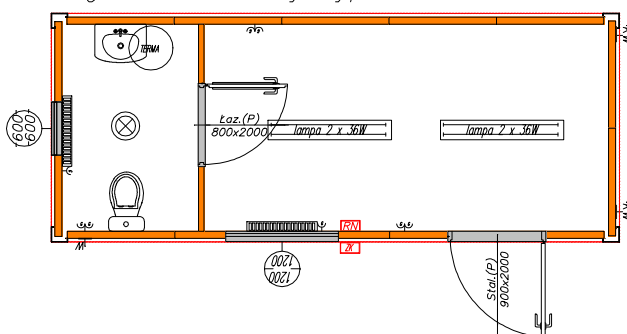
Segment biurowy typ 5
