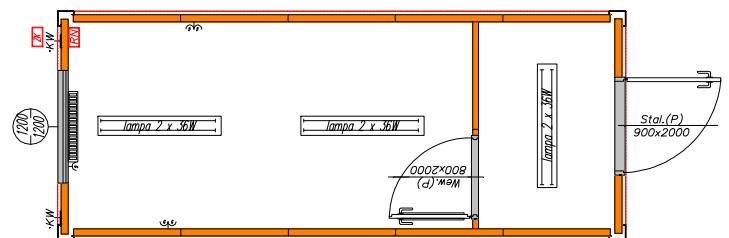
Segment biurowy typ 2
