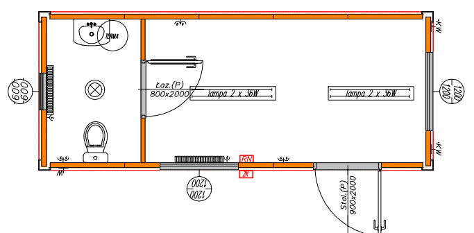
Segment biurowy typ 6
