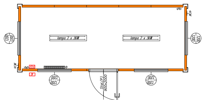
Segment biurowy typ 4
