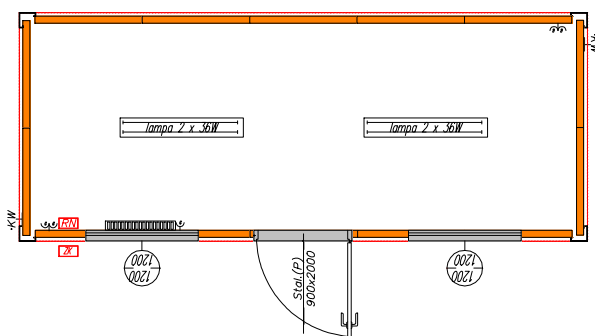
Segment biurowy typ 3
