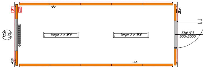
Segment biurowy typ 1
